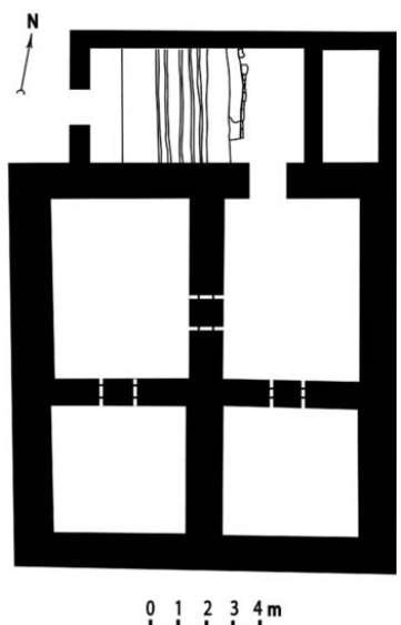
Іл. 18. План Мазепиного палацу на Гончарівці за археологічними дослідженнями його фундаментів. Реконструкція Ю. Ситого, комп'ютерна графіка С. Дмитрієнка.
