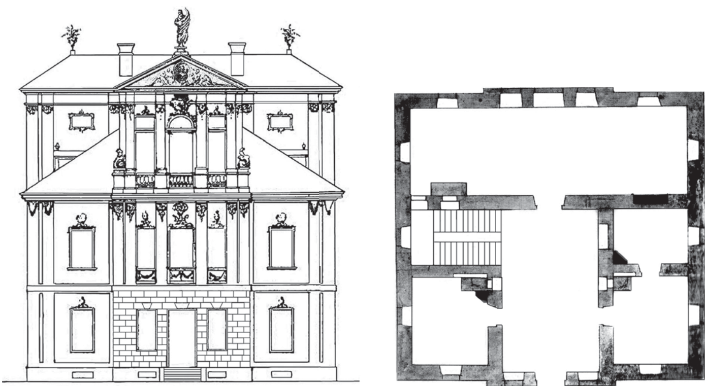
Іл. 17. Кресленики Т. Гамерена чільного фасаду з ризалітом та плану палацу Котовських у Варшаві 1684 р.
